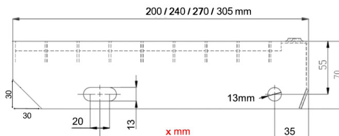
Bohrschema Seitenplatten Treppenstufen
