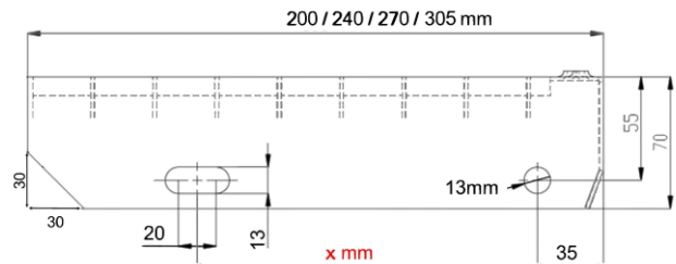
Bohrschema Seitenplatten Treppenstufen
